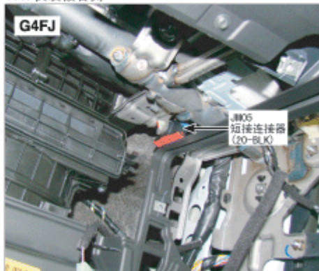
171. 仪表板右侧
