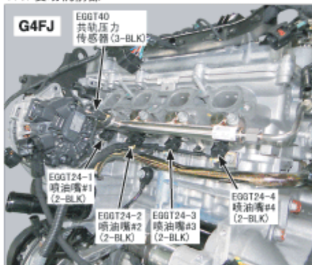
173. 发动机前部
