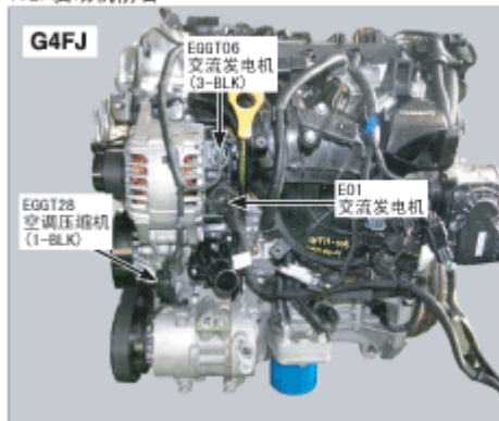
172. 发动机前右
