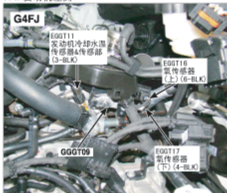
174. 发动机左侧
