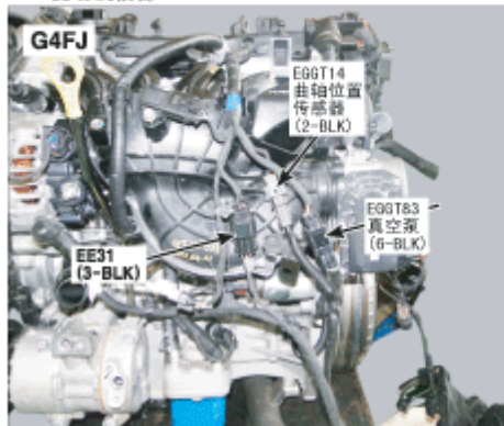
169. 发动机前部
